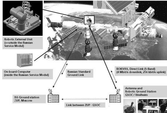
Fig. 5 System overview of ROKVISS
