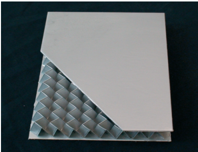
Aluminium Sandwich mit gefalteter Kernstruktur
