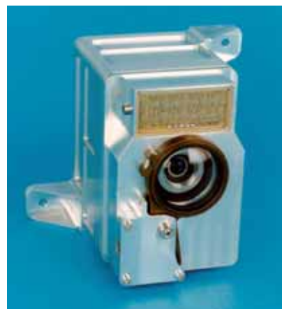
Die ROLIS-Kamera.
