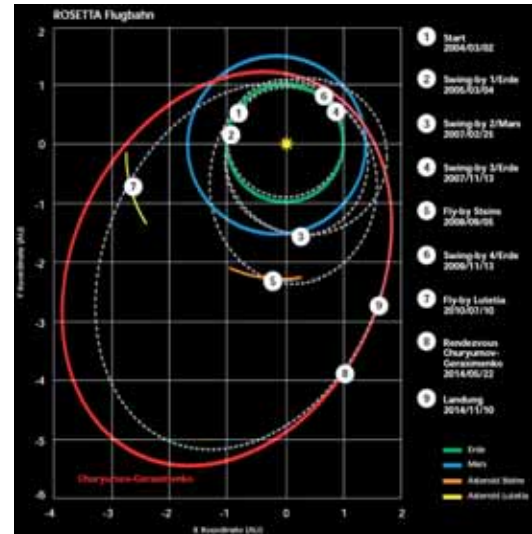
Rosettas Flugbahn durch das innere Sonnensystem.
