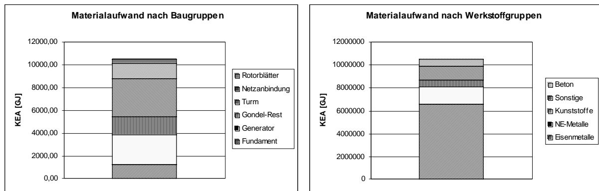
Abbildung 2.7: Energieaufwand für Baumaterial aufgeschlüsselt nach Bau- und Werkstoffgruppen
