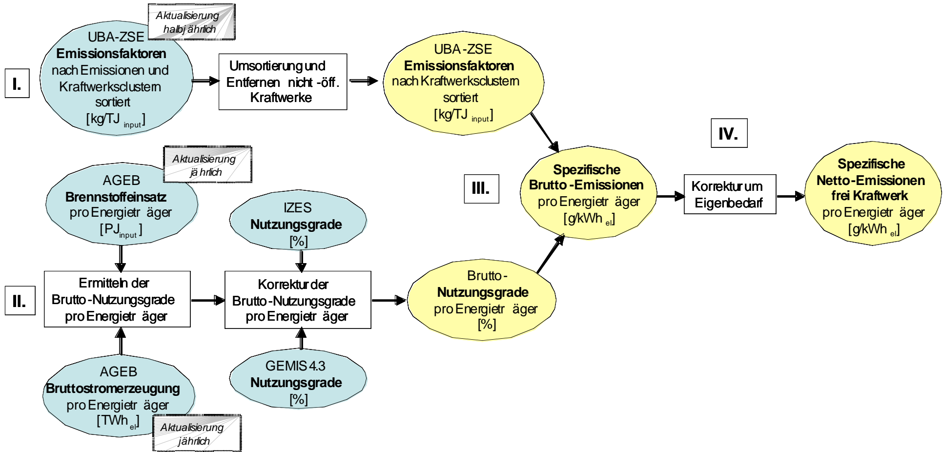
Abbildung 1.2: Rechenweg bei der Ermittlung der spezifischen Netto-Emissionen der fossilen Kraftwerke
