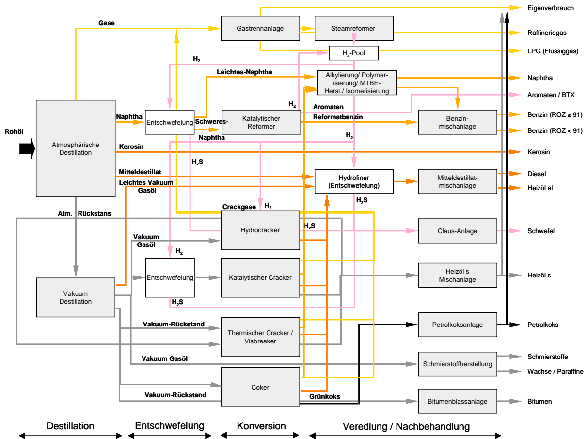
Abbildung 2.5: Vereinfachtes Verfahrensschaubild einer Raffinerie
