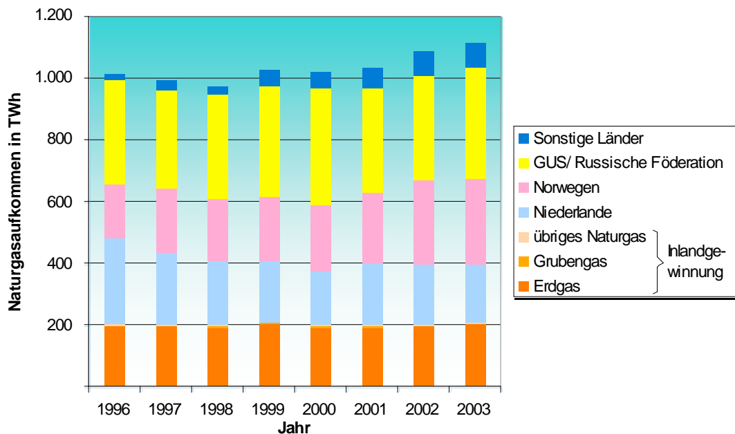
Abbildung 2.2: Zeitliche Entwicklung des Naturgasaufkommens in Deutschland
