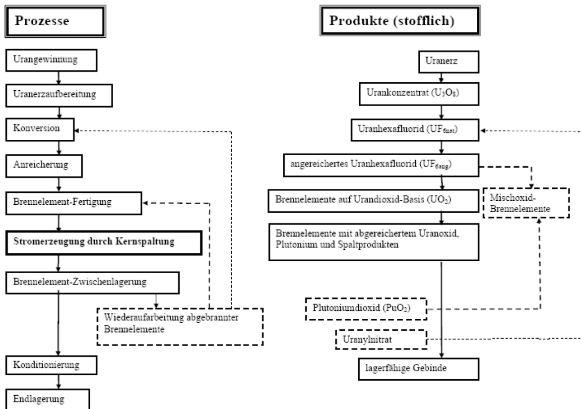
Abbildung 2.6: Brennstoffbereitstellung
