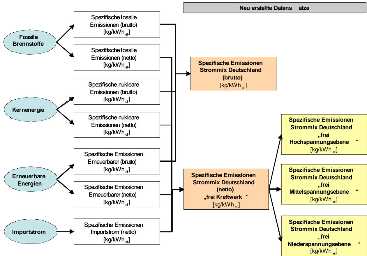
Abbildung 1.1: Rechenweg zur Erstellung der Grunddatensätze für den „Strommix Deutschland“ (nur direkte Emissionen)
