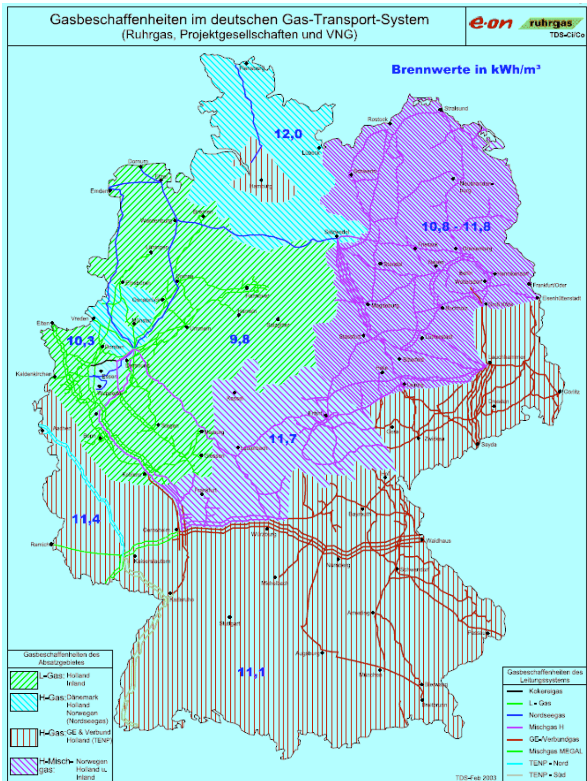
Abbildung 2.4: Gasbeschaffenheit im deutschen Gas-Transportsystem
