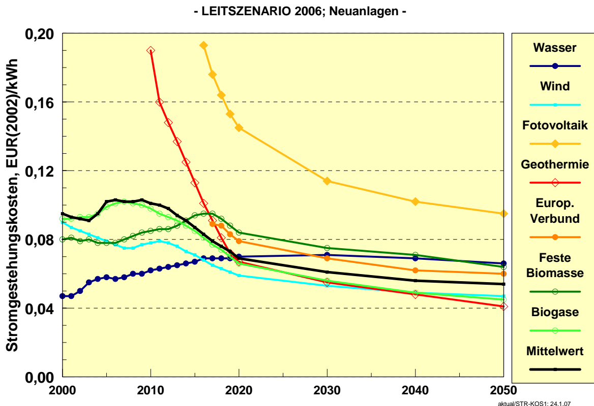
Bild 3: Zukünftige Kostenentwicklung der stromerzeugenden EE-Technologien bis 2050 und des Mittelwerts des gesamten EE-Mixes im LEITSZENARIO 2006, (Geldwert 2002; realer Zinssatz 6%/a; jeweils Mittelwerte mehrerer Einzeltechnologien)
