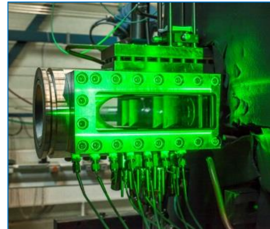
Eine optische Versuchsbrennkammer zur visuellen Analyse der Zündprozesse.
