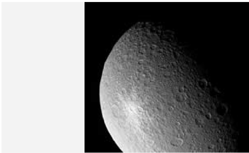
Oberfläche des Saturnmondes Rhea
