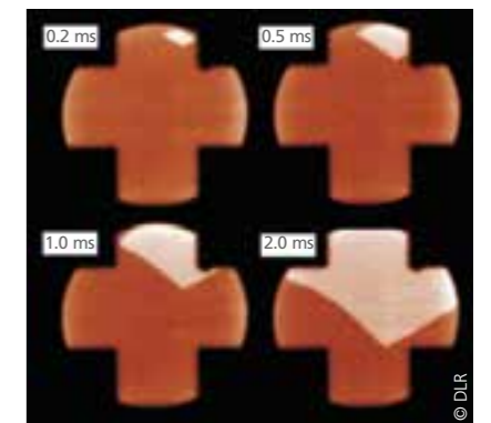
Die Erstarrungsfront einer Metalllegierung breitet sich von einem Punkt aus. The solidification front of a metal alloy propagates from one single point.
