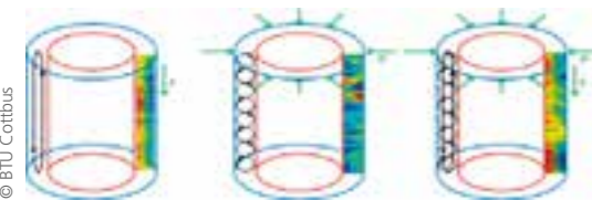
Schematische Darstellung der konvektiven Strömungen im Zylinderspalt (v. l.): natürliche Auftriebskonvektion unter Schwerkraft, thermische Konvektion unter Mikrogravitation, Überlagerung von thermischer und Auftriebskonvektion unter Erdschwerebedingungen
