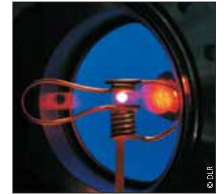
Bodenlevitation einer metallischen Legierung während des Schmelzens Ground levitation of a metal alloy sample during melting
