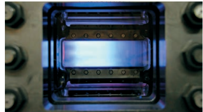
Blick in die gläserne Brennkammer des Hochdruckprüfstands mit FLOX®-Brenner in Betrieb
