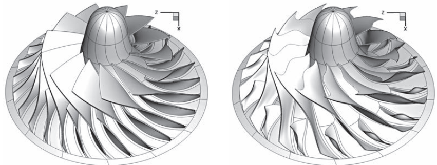
Optimierung eines Radialverdichters mit AutoOpti: Ausgangsgeometrie und eine der besten neuen Geometrien
