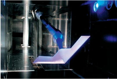
Hochgeschwindigkeitsmodell DLR-F17E im transsonischen Windkanal: Druckverteilungsmessungen mittels drucksensitiver Farbe
