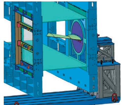
Konstruktion des Versuchsaufbaus des Flügels im TWG Göttingen
