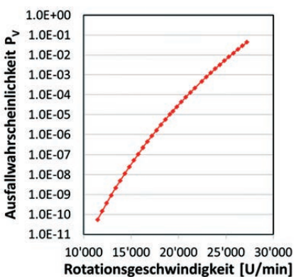
Ausfallwahrscheinlichkeit der Turbinenschaufel als Funktion der Rotationsgeschwindigkeit
