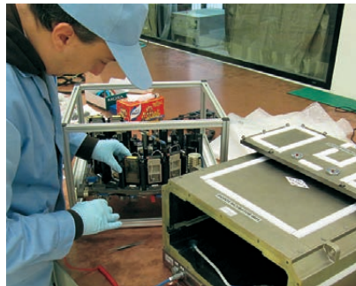
SIMBOX beim „Matching Test“ im Labor der GESSA in Peking: Die Zentrifuge wird in den Inkubator eingebaut
