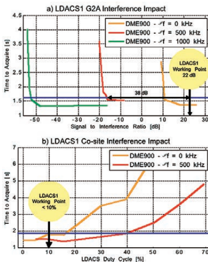
Interferenzeinfluss von LDACS1 auf DME beispielhaft für das DME-System DME900 von Rockwell Collins:
