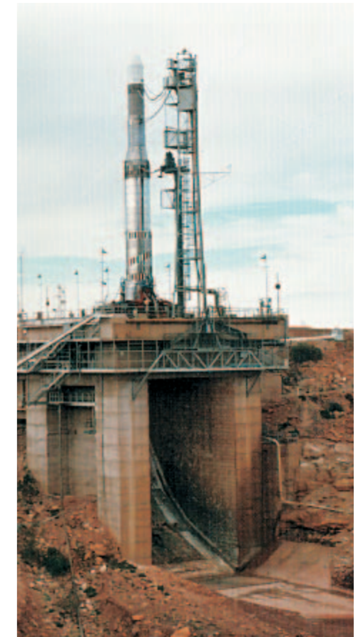
Die Europa 1-Rakete war die erste einer Serie europäischer Trägerraketen aus den 1960er- und 70er-Jahren. Sie wurde von der ELDO (European Launcher Development Organisation) entwickelt. Testflüge starteten in Woomera, Australien (ca. 1970).
