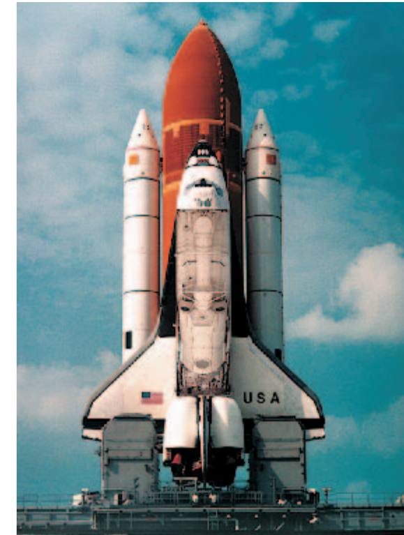
28. September 1983: „Röntgenblick“ auf das Spaceshuttle Columbia. Innenliegend das Spacelab (unten), darüber der Verbindungstunnel zum Cockpit.
