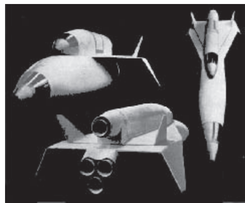
Entwürfe von Sänger I (Bild links: Junkers) und Sänger II (Bild unten: MBB/EADS) Blueprints of Sänger I (left, picture: Junkers), Sänger II (below, picture: MBB/EADS)
