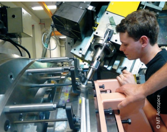
Zur Herstellung der Oberstufentanks für die Ariane 5ME kommt im europäischen Raumtransport erstmals das „Reibrühr-schweißverfahren“ zum Einsatz. Dieses effiziente und materialschonende Verfahren hat auch in der Raumfahrt ein erhebliches Zukunftspotenzial.
