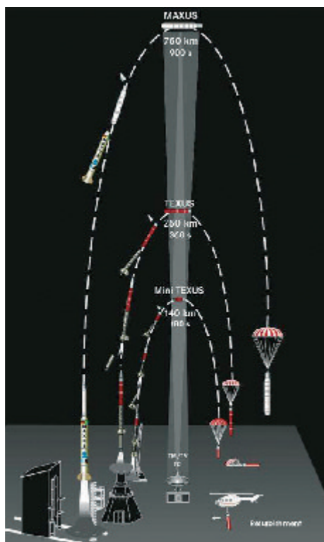
Schematische Darstellung der Texus-Flugparabel im Vergleich mit anderen Höhenforschungsraketen (EADS Astrium)
