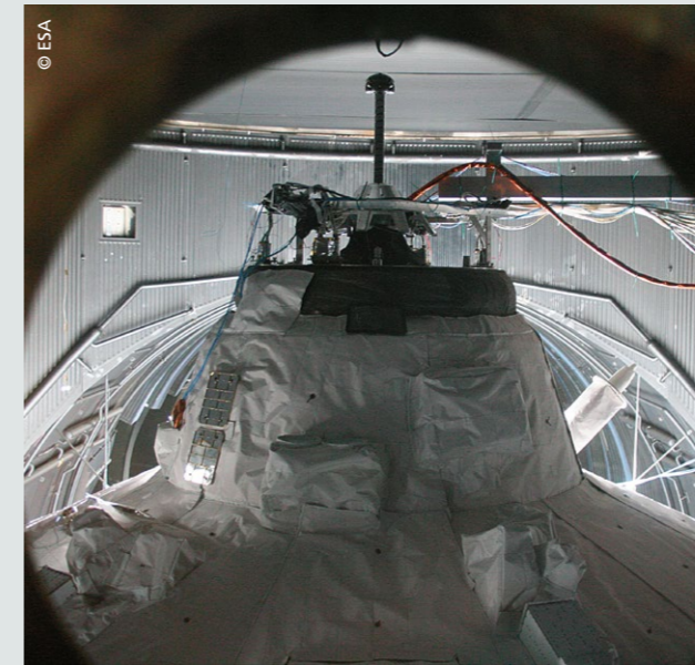
Der ATV-Dockingmechanismus ist eine hochkomplexe Angelegenheit: Ein Drehstab am Ende des ATV-Dockingmoduls gleitet beim Ankoppeln in das Dockingmodul der ISS und zieht das Raumschiff an die ISS heran. Über mehrere Bolzen und Haken wird dann eine dichte Verbindung hergestellt.
