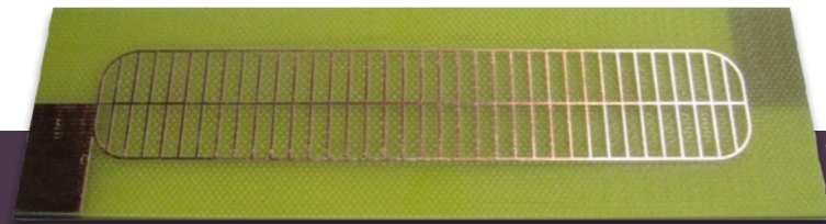
Verbesserte Elektroden zur Erzeugung des Plasmas. Ein Rahmen um die kammähnlichen Spitzen verhindert Erosionsschäden an der Leiterplatte.
