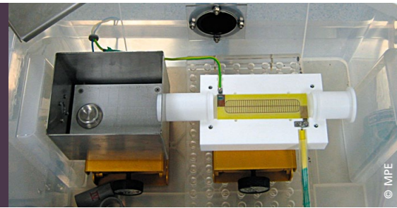
KAP-Bestrahlungsvorrichtung zur Dekontamination von Raumfahrtbauteilen
