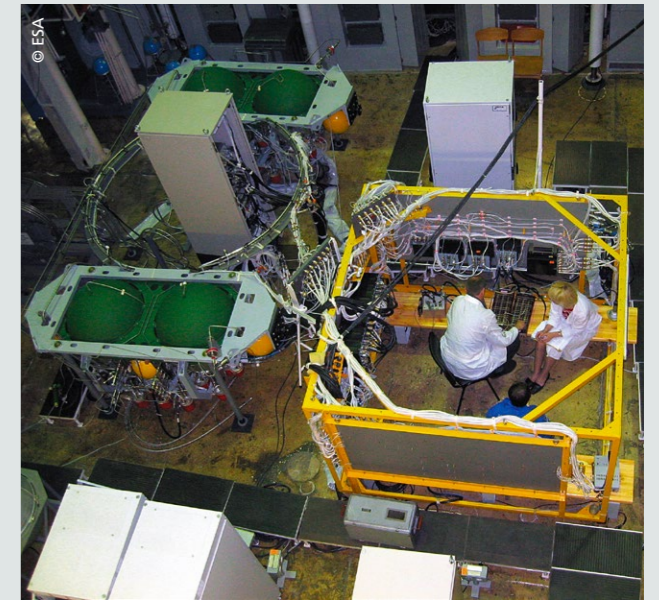
Das russische „Equipment Control System“ wird bei RSC-Energia in Korolyov in der Nähe von Moskau hergestellt. Dieses Kontrollsystem wird in das druckbeaufschlagte Transportmodul des ATV-1 „Jules Verne“, das an die ISS andockt, eingebaut. In 20 Transportboxen wurde das System zum ESA-Standort ESTEC in Noordwijk verschifft, wo es mit Hilfe von russischen Ingenieuren in das erste ATV-Flugmodell eingesetzt wurde.
