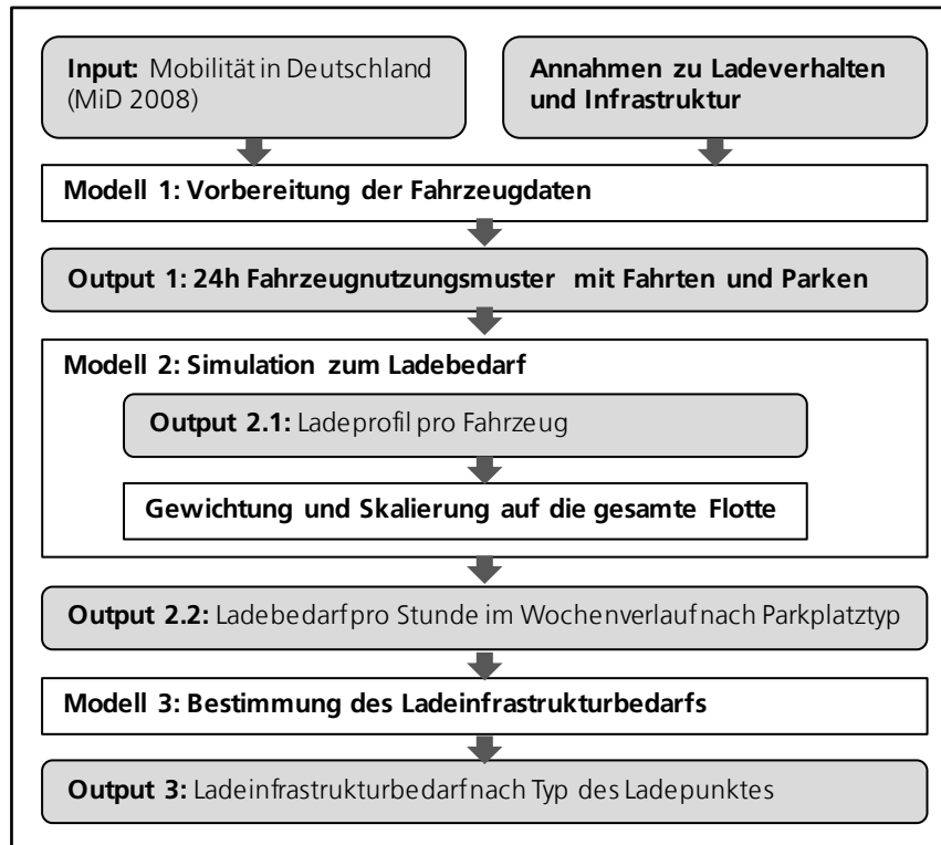
Abbildung 4: Übersicht der Methodik zur Bestimmung von bedarfsgerechter Ladeinfrastruktur, wie im Current -Modell implementiert (MiD: 2008 Mobilität in Deutschland).
