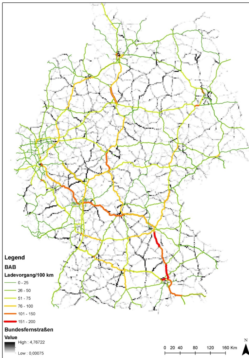
Abbildung 9: Ladevorgänge im Fernverkehr als Dichte (Ladevorgang pro 100 km Streckenabschnitt). Ladevorgänge auf Bundesfernstraßen werden in Rasterzellen dargestellt, dabei bilden schwarze Zellen eine hohe und graue Zellen eine entsprechend niedrigere Anzahl von Ladevorgängen ab.
