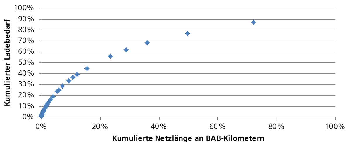
Abbildung 10: Verteilung des Ladebedarfs auf das Autobahnnetz in Deutschland.
