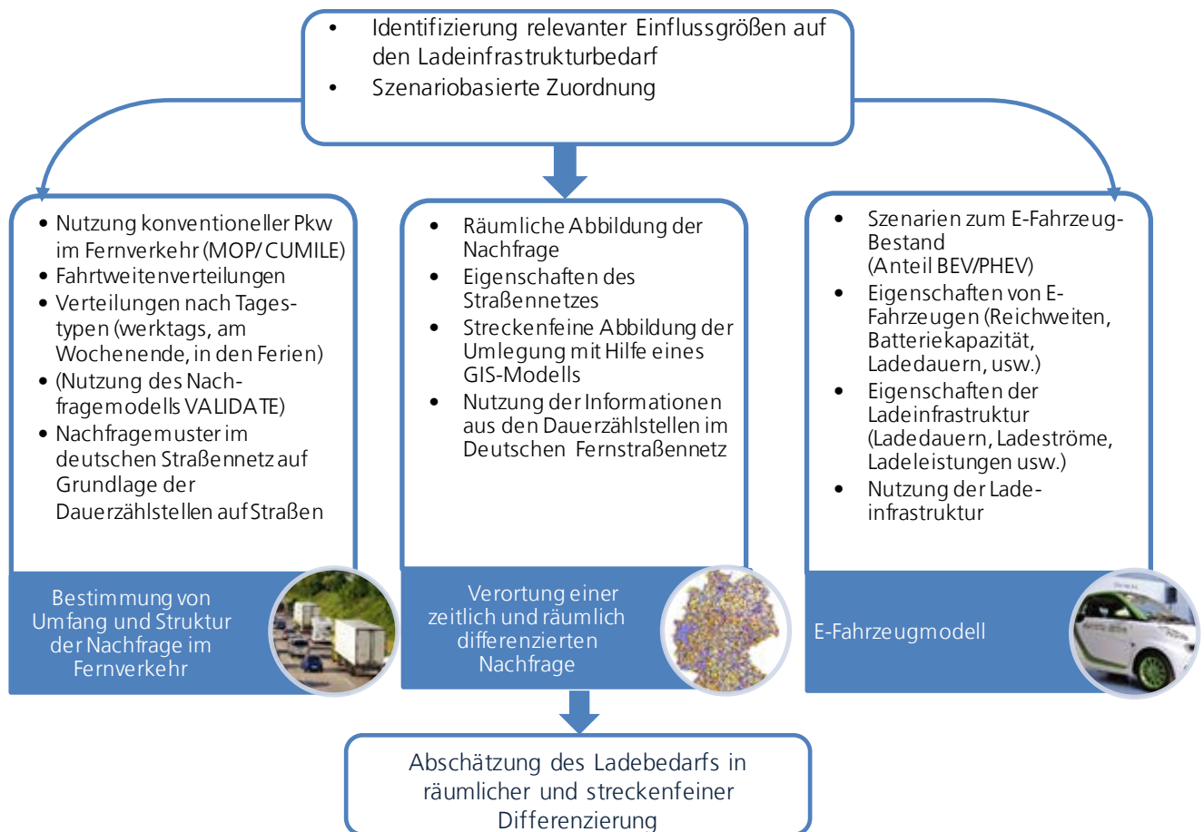
Abbildung 8: Gesamtmodellübersicht zur Abschätzung des Ladeinfrastrukturbedarfs im Fernverkehr.
