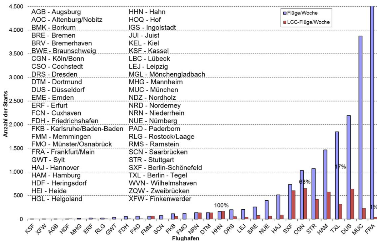
Abbildung 3: Angebotene Passagierflüge pro Woche auf deutschen Flughäfen im Juli 2016 (ohne Air Berlin)
