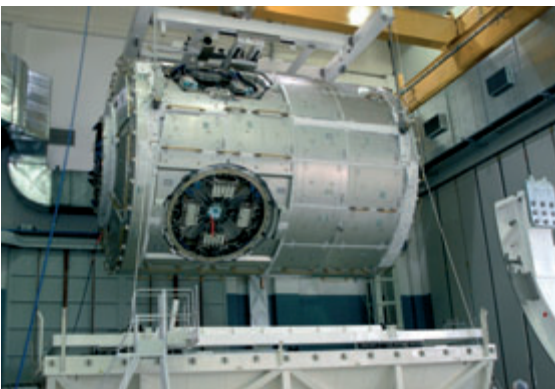
Der europäische Verbindungsknoten 2 zum Andocken von COLUMBUS und KIBO
