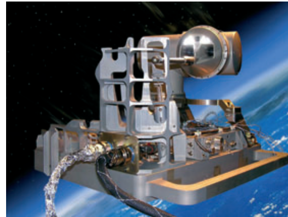
Roboterarm ROKVISS im Weltraum The ROKVISS Robotic Arm in Space
