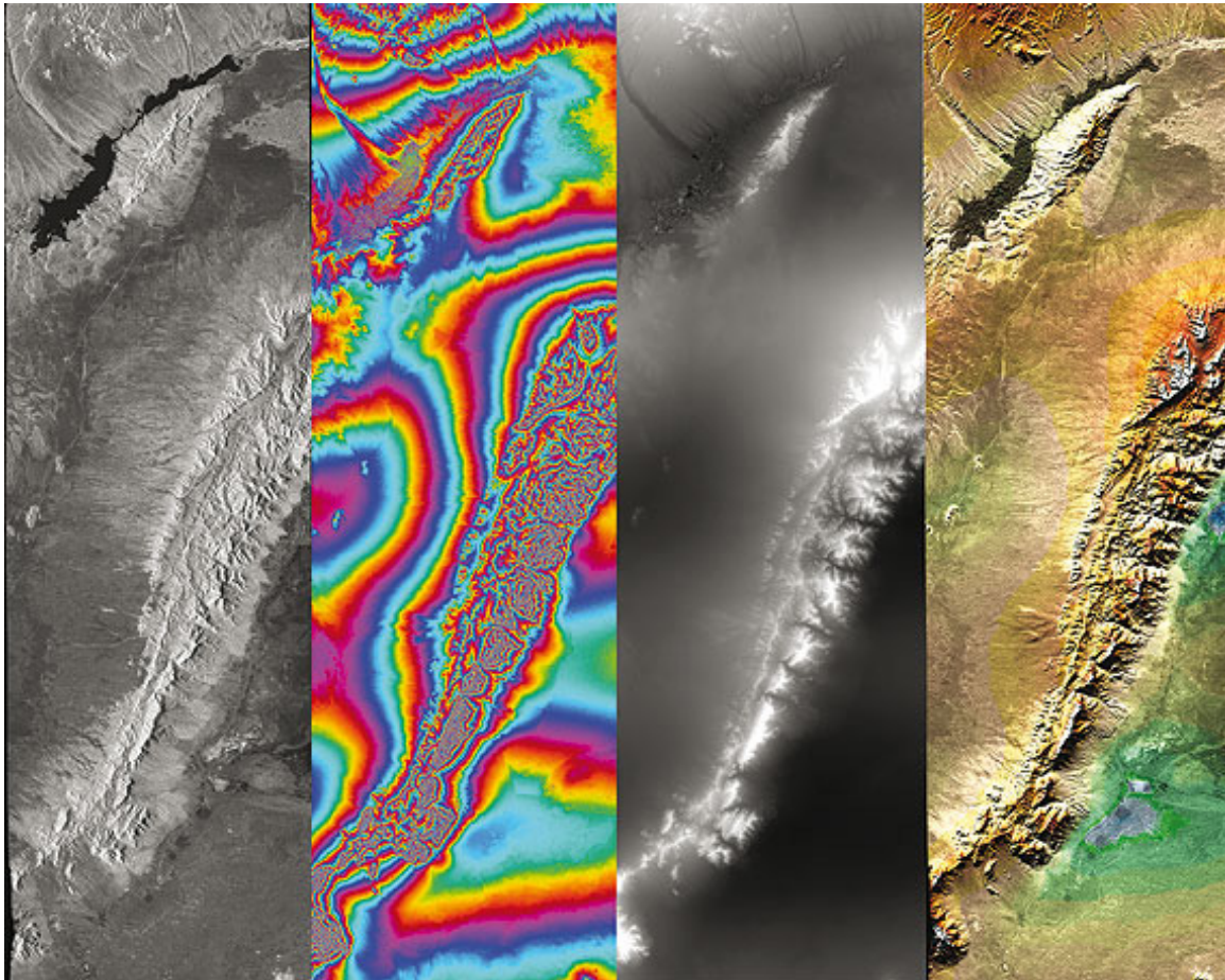
Darstellungsformen der SRTM-Daten
