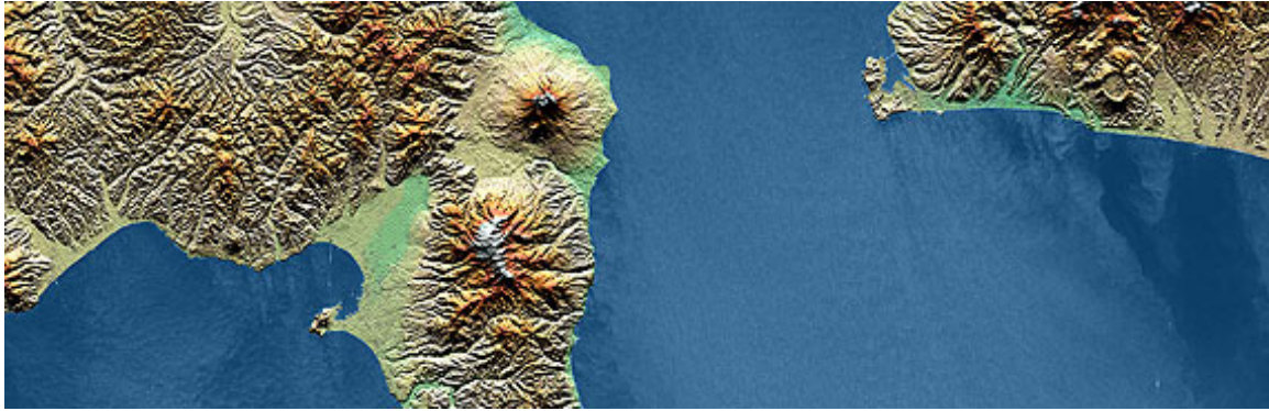
SRTM-Aufnahme von Hokkaido
