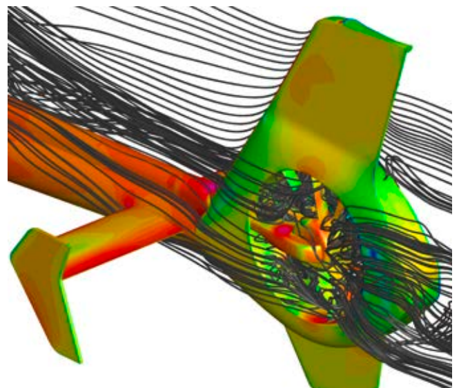
Stromlinien und Druckverläufe bei einem Airbus Helicopters EC135 Fenestron
