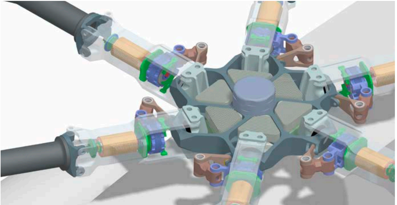
Rendering des 3D-Modells der Taumelscheibenlosen Blattwurzelsteuerung aus unseren Projekten InHuS und ELBA.
