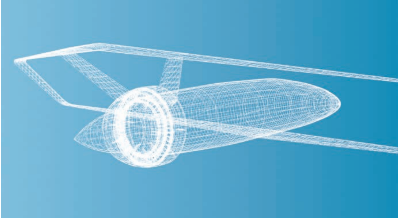
„Propulsive Fuselage“-Konzept aus dem Bauhaus Luftfahrt in München: Die interdisziplinäre Forschungseinrichtung untersucht eine Verteilung der Schubproduktion eines Flugzeugs um den gesamten hinteren Rumpf herum. Dies könnte eine optimale Basis für die Nutzung der so genannten Grenzschichteinsaugung darstellen, mit deren Hilfe der Widerstand des Flugzeugrumpfes signifikant reduziert werden könnte.
